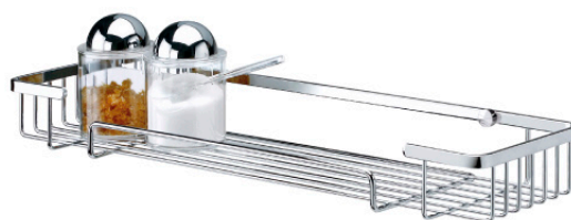
HC-5329-1450 多功能置物架 Multipurpose Rack L520 x W140 x H60 mm (附 HC-5701 螺絲帽組)
